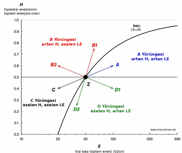
Şekil 1: Hiyerarşik-Enerji Alanında Yörüngeler
